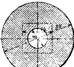
Фиг. 6. Разръзъ по gh .
