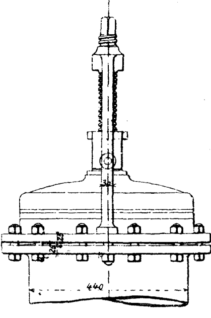
Фиг. 14. Боковой видъ.
