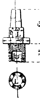
Фиг. 12. Фреза.
