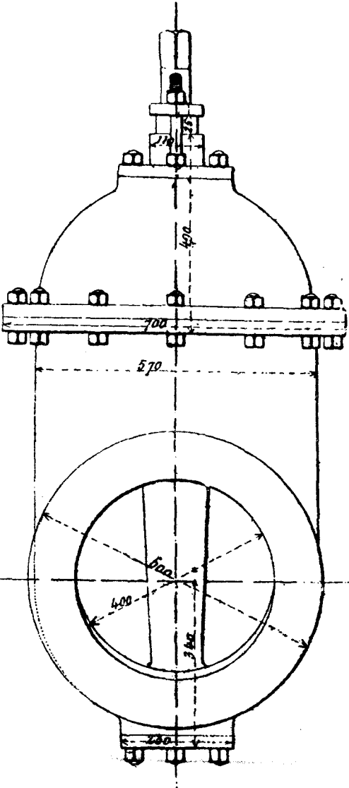
Фиг. 4. Боковой видъ.
