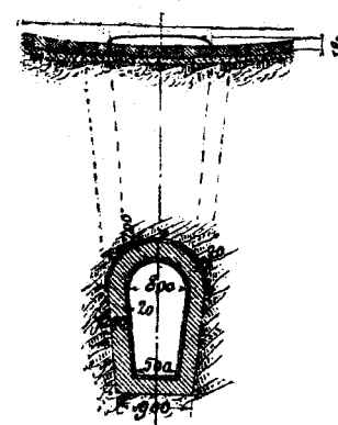
Масштабъ фиг. 2, 3, 4, 5 : 1/100.
