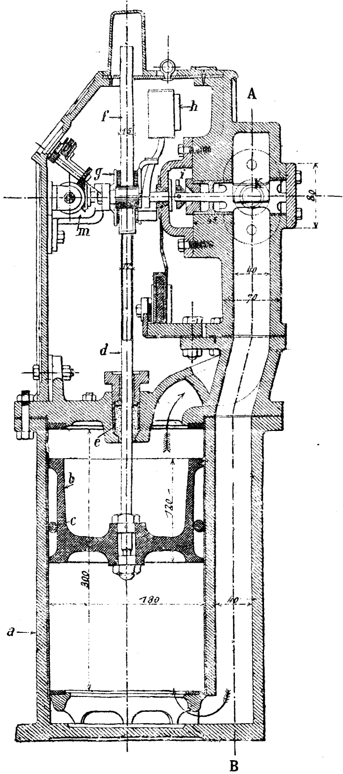
Фиг. 2. Разрѣзъ по CDEF.
