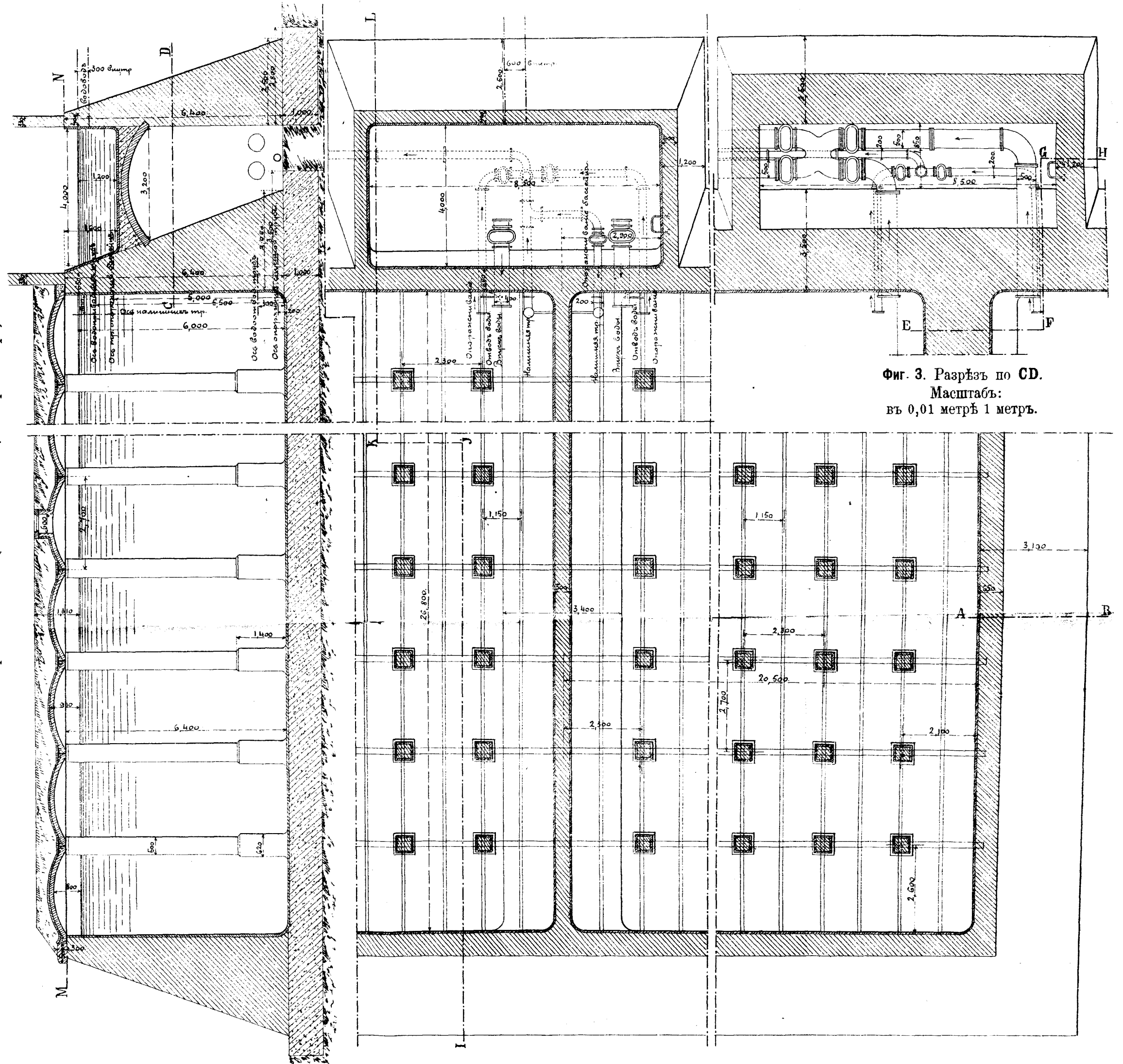
Фиг. 2. План и разрез по MN Масштаб: въ 0,01 метрѣ 1 метрѣ.
