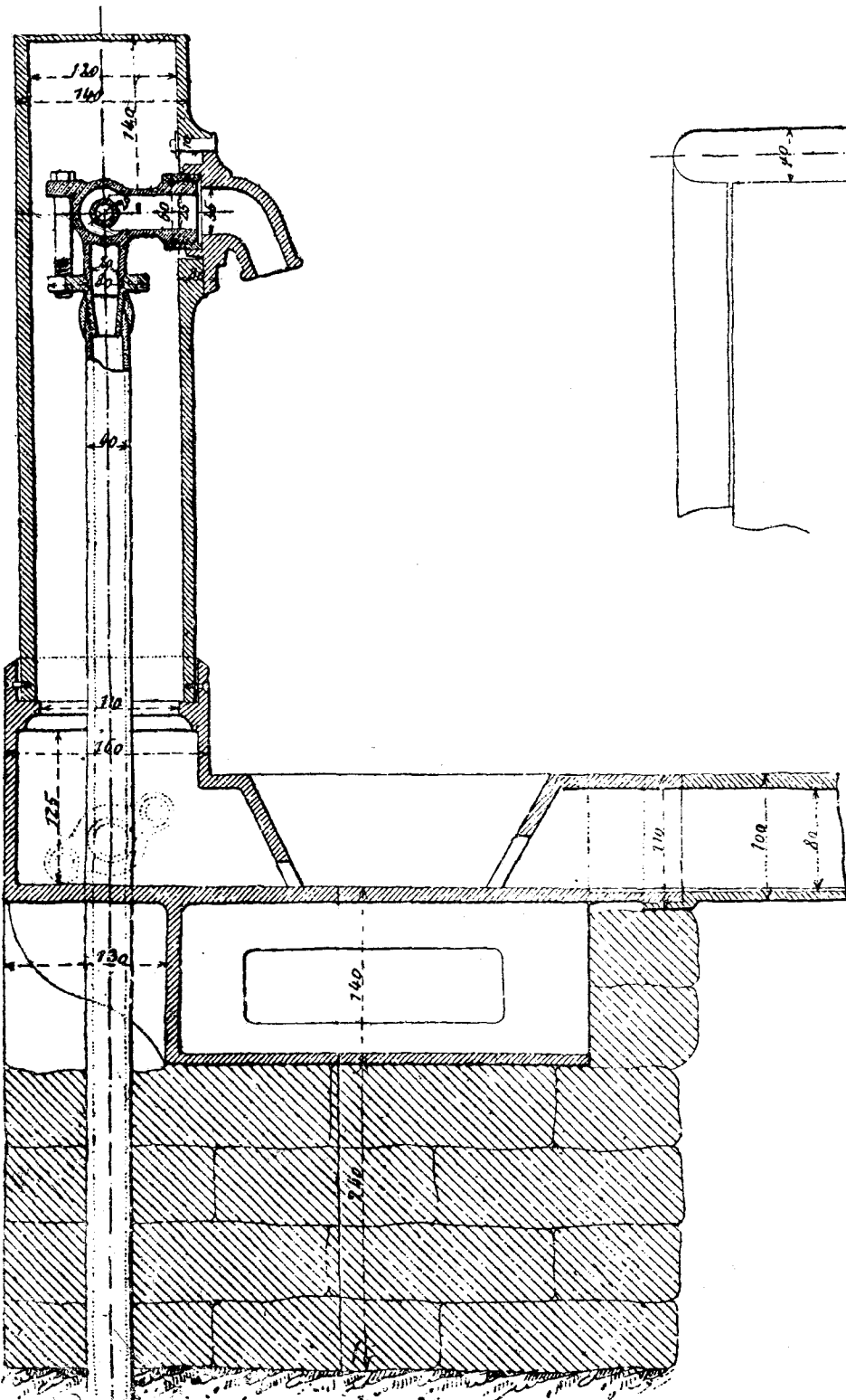
Фиг. 2. Поперечный разръзъ.
