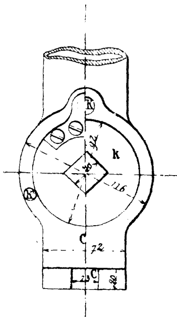
Фиг. 8. Кранъ.
