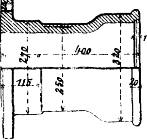
Фиг. 6. Разрѣзъ и горизонтальная проекція.
