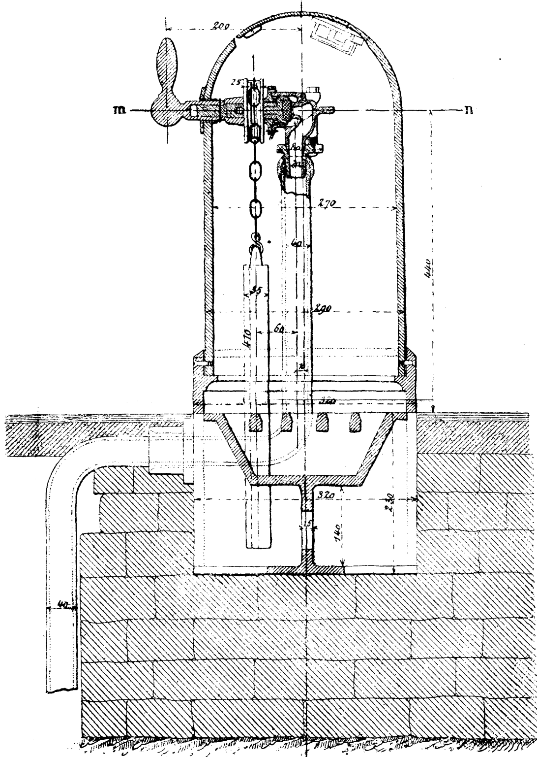
Фиг. 1. Продольный разръзъ.
