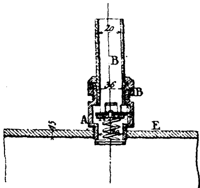
Фиг. 1. Вертикальный разръзъ отвьтвленія (вмѣстѣ съ главной трубой).
