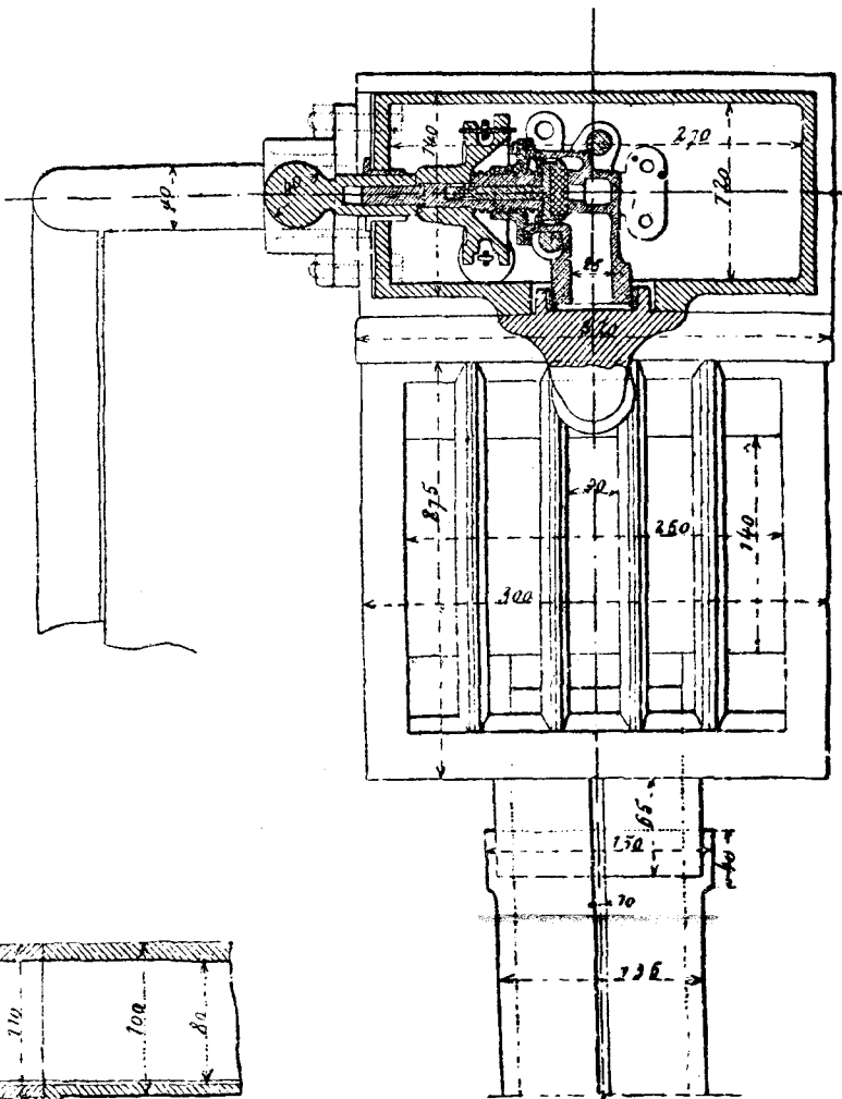
Фиг. 3. Планъ и разръзъ по mn .
