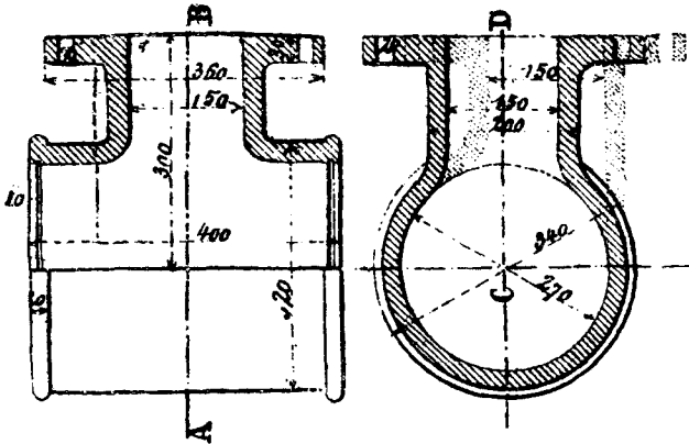
Фиг. 7. Разрѣзъ по ED.
