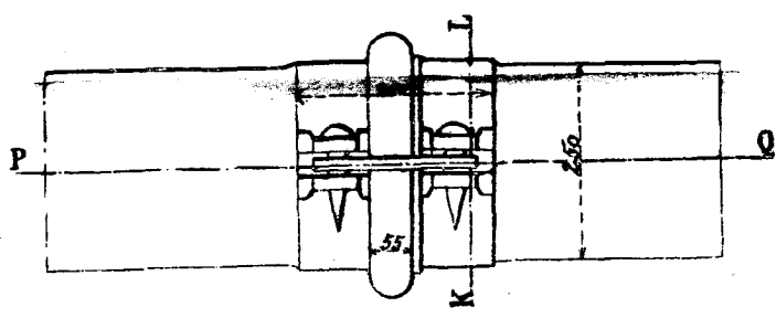
Фиг. 13. Видъ сверху.
