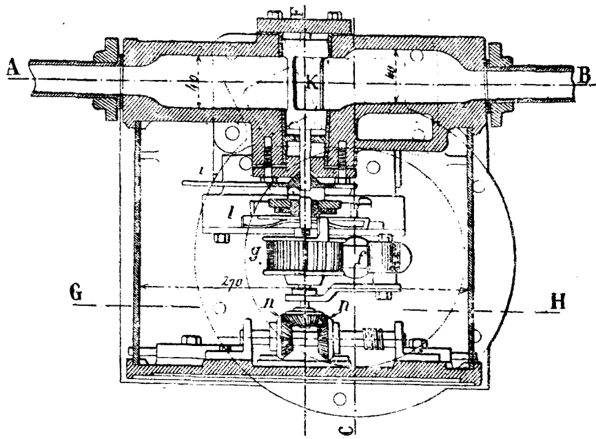
Фиг. 4. Планъ.
