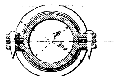
Фиг. 14. Разрѣзъ по KL.
