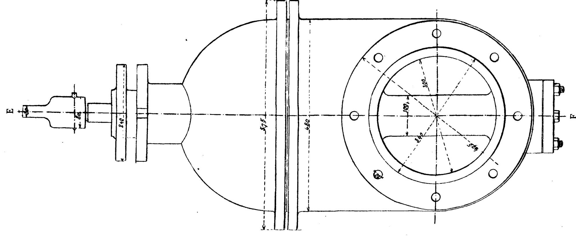
Фиг. 4. Планъ.
