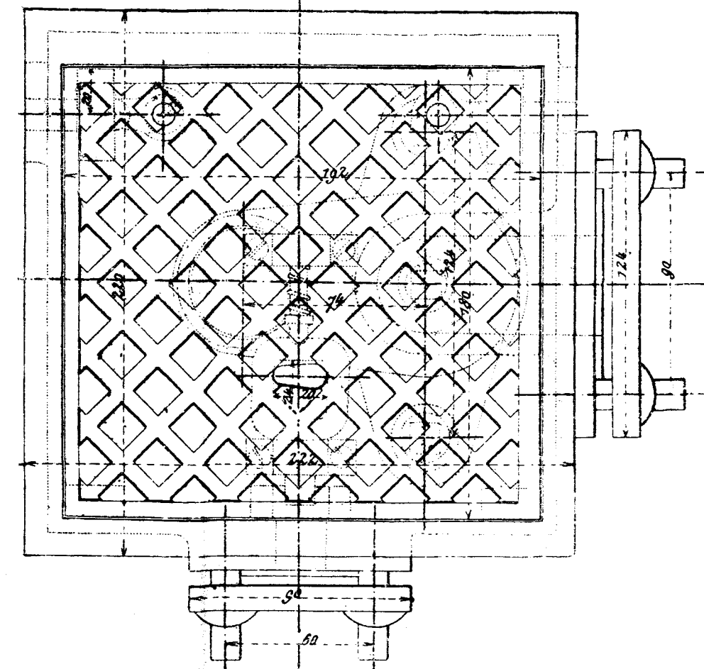
Фиг. 4. Планъ.
