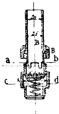
Фиг. 2. Вертикальный разръзъ отвьтвленія (отдѣльно отъ главной трубы).
