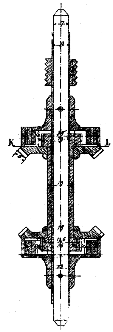
Фиг. 4. Разрѣзъ по MN (безъ счетныхъ колесъ).
