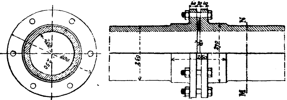
Фиг. 3. Разрѣзъ по MN.
