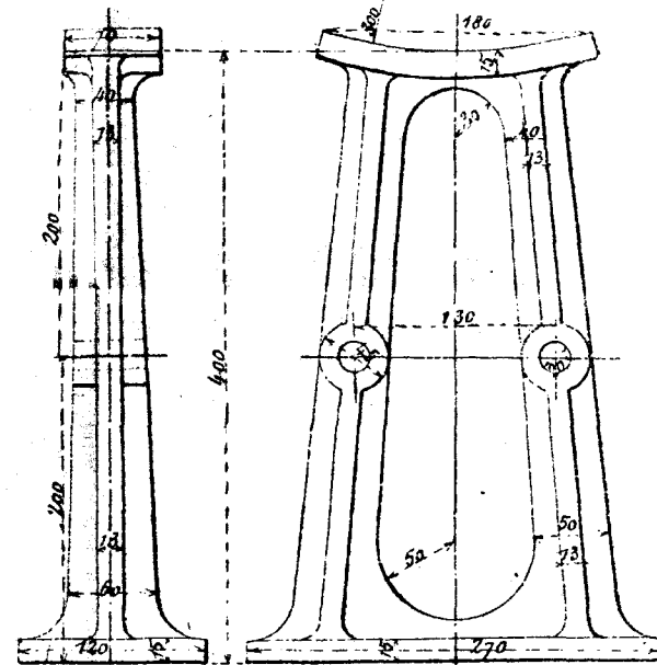
Подставка для створнаго крана отъ 0,12—0,30 метра. Фиг. 6. Боковой видъ. Фиг. 7. Передній видъ.
