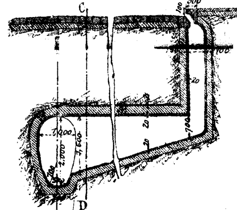
Поперечный разръзъ канала № 6 и уличнаго водоспуска.
