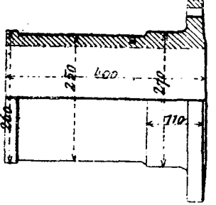
Фиг. 5. Разрѣзъ и горизонтальная проекція.
