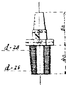
Фиг. 11. Мѣтчикъ.
