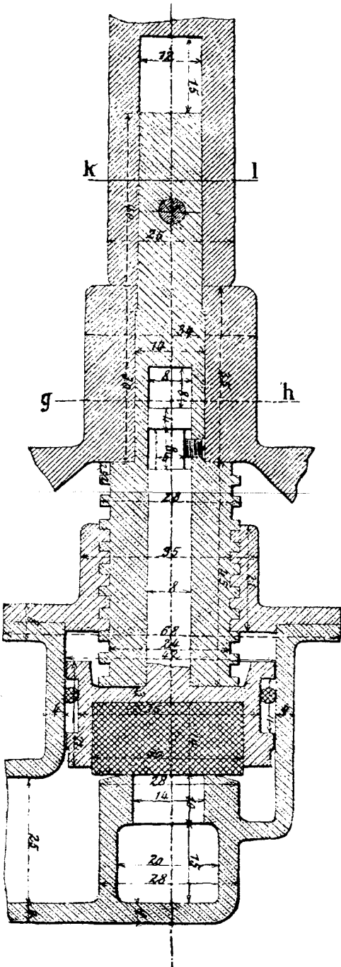
Фиг. 4. Разръзъ по mn (въ натуральную величину).
