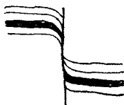
Фиг. 8. Сбросъ.
