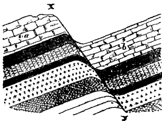
Фиг. 9. Сбросъ.
