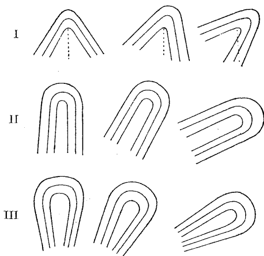
Фиг. 5. Типы складокъ.
