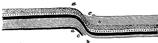
Фиг. 7. Флексура.
