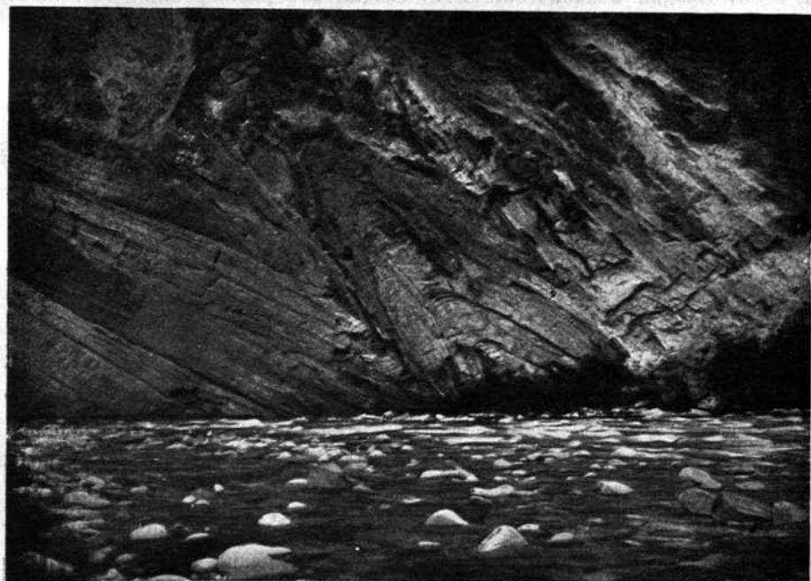
Фиг. 3. Обнаженіе кристаллическихъ сланцевъ на берегу р. Олекмы. Кристаллическіе сланцы (филлиты) собраны въ средней части обнаженія въ небольшую наклонную, нормальную, антиклинальную складку, ограниченную съ обѣихъ сторонъ ненормальными сбросами (взбросами).
