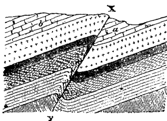
Фиг. 10. Взбросъ.
