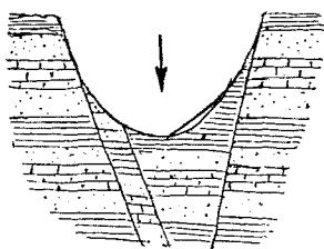
Фиг. 13. Грабенъ.
