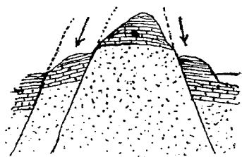
Фиг. 14. Гореть.
