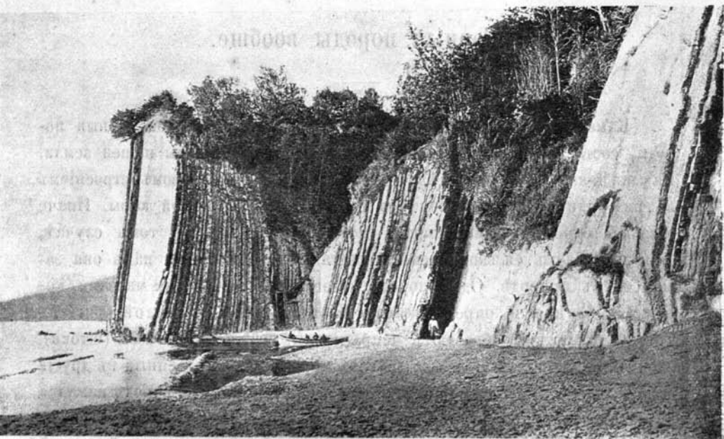
Фиг. 1. Пласты мергелей, поставленные почти на головы. Берегъ Чернаго моря около Туансе.
